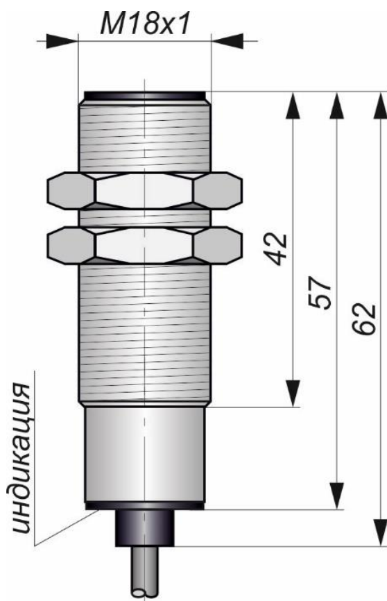
Габаритный чертеж
